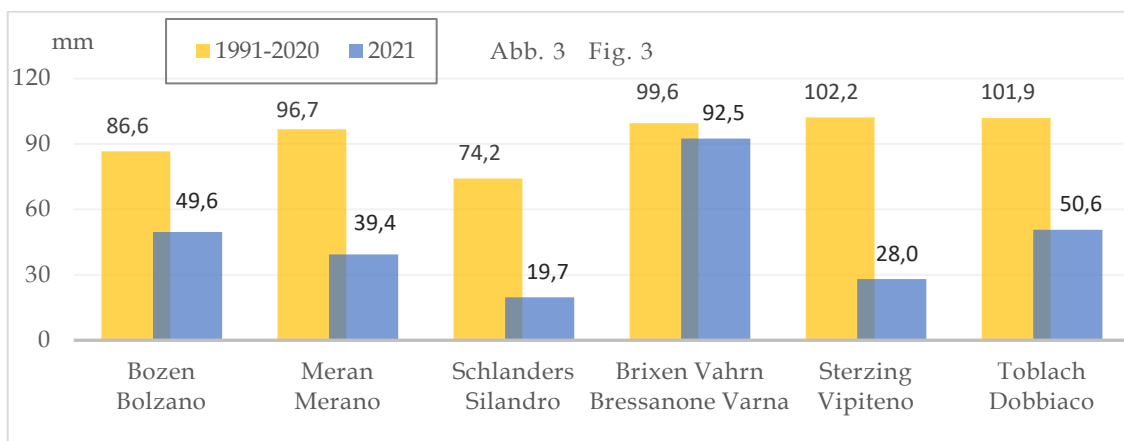
Abb. 3: Monatliche Niederschlagssummen (blau), Mittelwert der Periode 1991-2020 (gelb): Im Juni gab es schon einige heftige Gewitter, die sorgten aber nur lokal für ergiebige Niederschläge. Südtirolweit gesehen war es dagegen trockener als normal.
