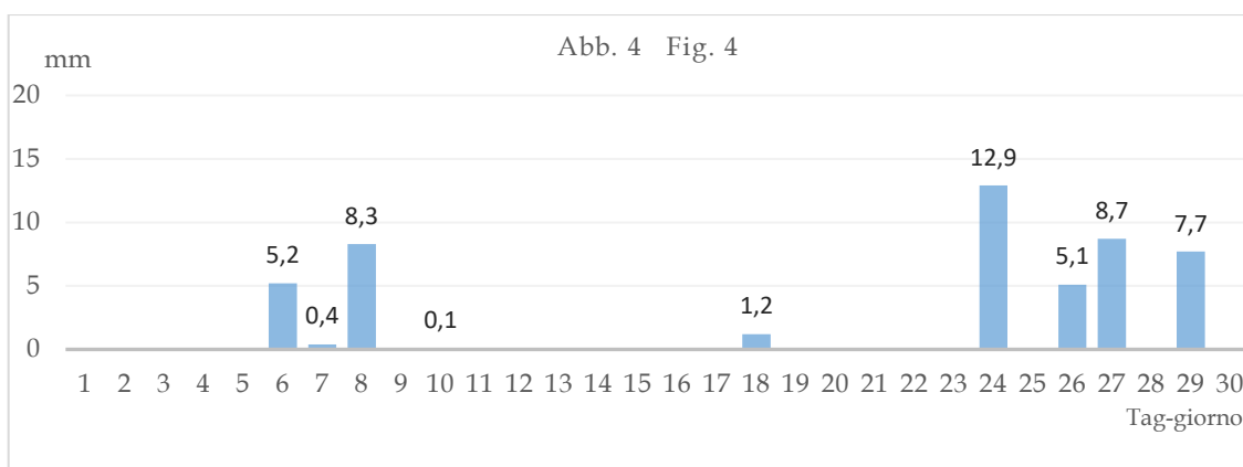
Abb. 4: Station Bozen, tägliche Niederschlagssummen (Zeitraum 09.00 Uhr MEZ des Vortages bis 09.00 Uhr MEZ des aktuellen Tages): In Bozen gingen im Juni mehrere starke Gewitter nieder, eines der stärksten mit Sturmböen ereignete sich am 23. Juni.
