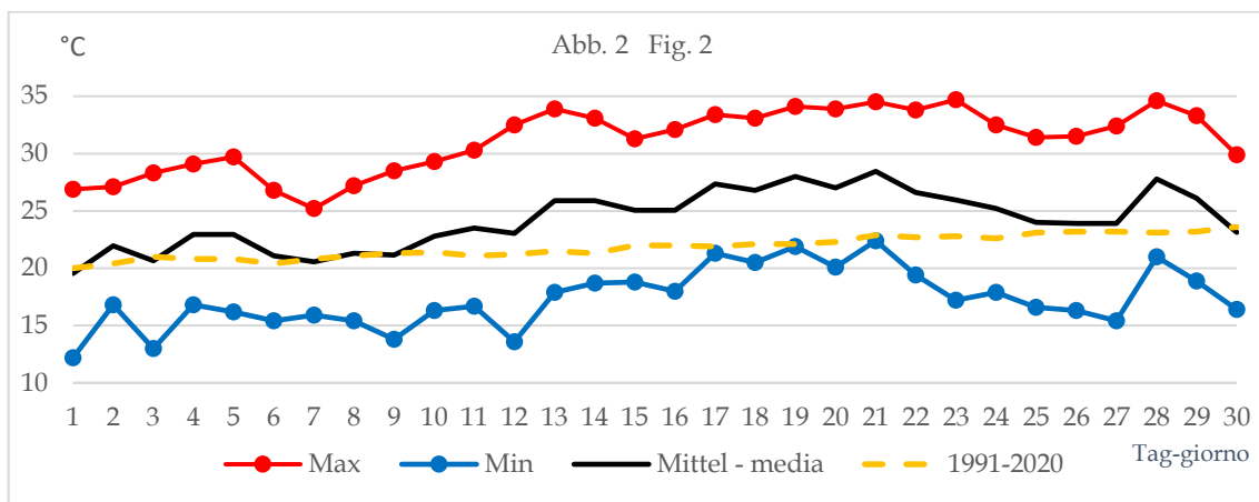
Abb. 2: Station Bozen: Tägliches Temperaturminimum (blau), -maximum (rot), Tagesmitteltemperatur (schwarz) und langjährige Tagesmitteltemperatur 1991-2020 (strichliert): Im Juni gab es zwar keine ausgeprägte Hitzewelle, aber durchgehend relativ hohe Temperaturen sowohl tagsüber als auch nachts.
