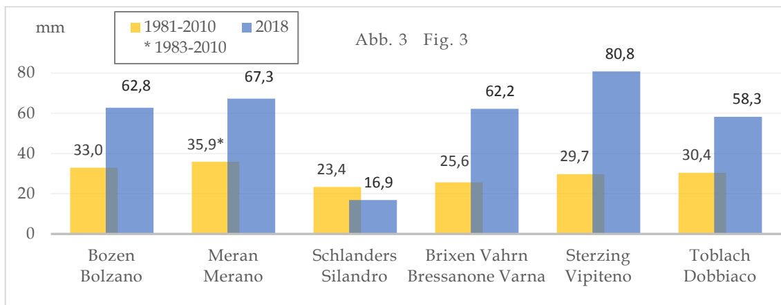
Abb. 3: Monatliche Niederschlagssummen (blau), Mittelwert der Periode 1981-2010 (gelb); Im Großteil des Landes verlief der März sehr nass, in vielen Landesteilen ist doppelt so viel Regen gefallen wie üblich. Lediglich im Vinschgau (Station Schlanders) regnet es weniger als üblich.
