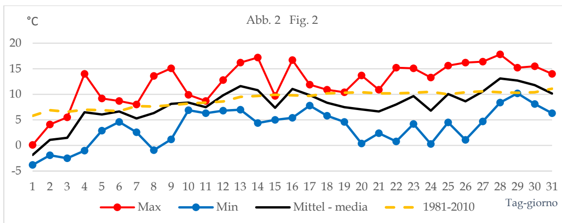
Abb. 2: Station Bozen. Tägliches Temperaturminimum (blau), -maximum (rot), Tagesmitteltemperatur (schwarz) und langjährige Tagesmitteltemperatur 1981-2010 (strichliert): Der März hat noch winterlich begonnenen, an den ersten beiden Tagen schneite es selbst in Bozen. Aber auch danach blieben die Temperaturen oft unterdurchschnittlich.
